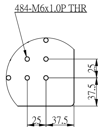
細部放大圖 A 比例 1:3
