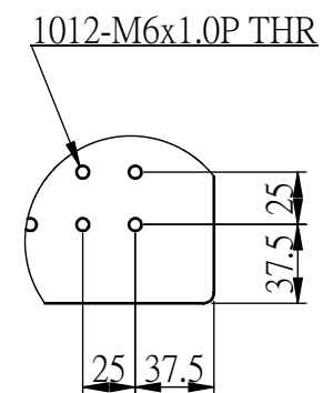
細部放大圖 A 比例 1 : 4
